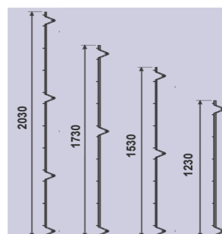
výšky panelů 3D
