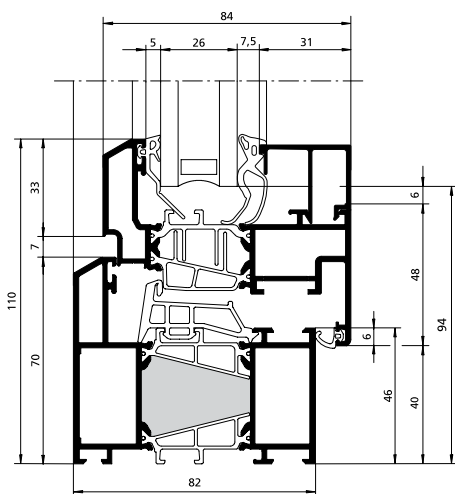
Řez profilem okna Heroal 090
