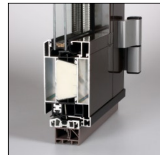
Heroal 090 - vstupní dveře
