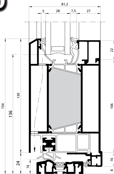
Řez profilem vstupních dveří Heroal 090
