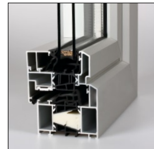
Heroal 090 - okno
