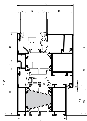
Řez profilem okna Heroal 110E
