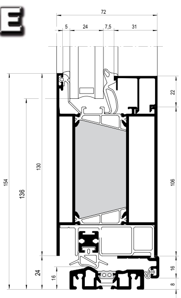
Řez profilem vstupních dveří Heroal 110E
